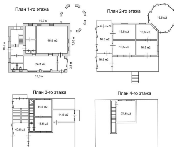
Рис.4. – Поэтажный план («Дача N5»)
